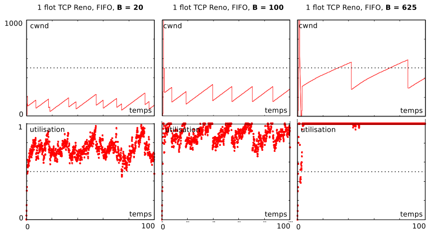
FIGURE 5.4 – Evolution de cwnd et utilisation de la bande passante disponible faite par une connexion TCP Reno en compétition avec une charge background de 50%, pour des tailles de buffer de 20, 100 et 625 paquets.
