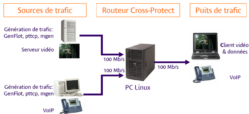
FIGURE 3.6 – Plateforme de démonstration Cross-Protect
