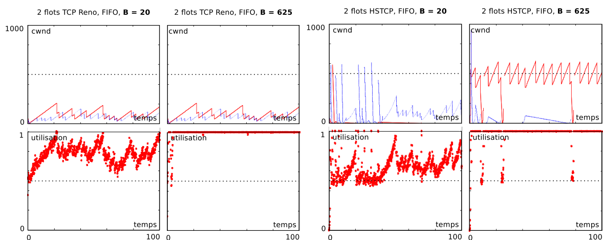
FIGURE 5.6 – Evolution de cwnd et utilisation de la bande passante disponible faite par deux connexions TCP Reno (à gauche) et deux connexions HSTCP (à droite), en compétition avec une charge background de 50%. Le lien est FIFO et les tailles de buffer de 20 et 625 paquets.
