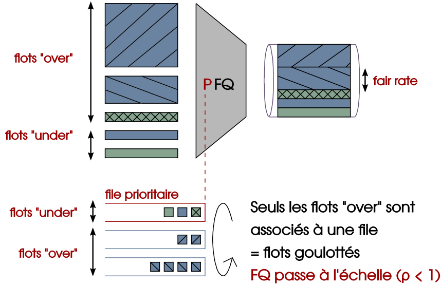
FIGURE 3.4 – Illustration du fonctionnement de l'algorithme PFQ
