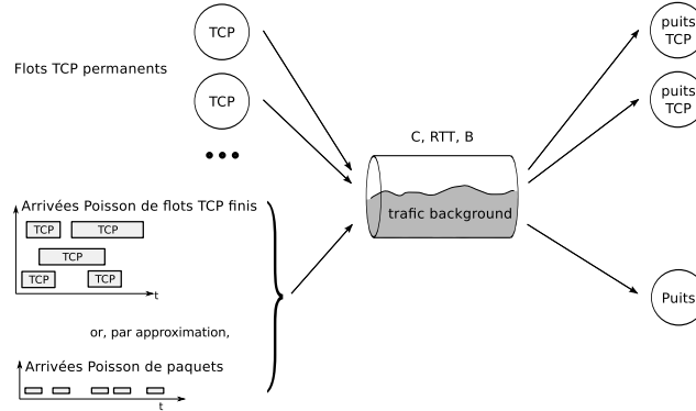
FIGURE 4.3 – Environnement de simulation : sauf précision supplémentaire, les simulations utilisent les paramètres suivants : C = 50\text{ Mb/s} , B = 20 paquets, RTT = 100\text{ ms} , \rho_b = 0.5C , ordonnancement FIFO, paquets de 1000 octets.
