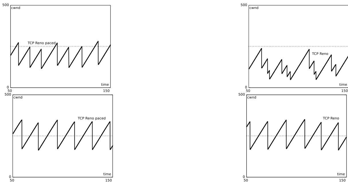
FIGURE 5.20 – Evolution de cwnd pour un flot Reno avec pacing (à gauche) et un flot Reno sans pacing (à droite), pour des tailles de buffers B = 20 paquets (en haut) et B = 100 paquets (en bas), pour C = 50 Mbps, \rho_b = 0.5
