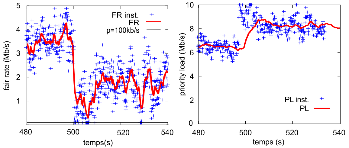
FIGURE 6.7 – Evolution du fair rate (à gauche) et du priority load (à droite) lors d'un événement de flashcrowd avec MinVar, k = 2 , p = 100\text{kb/s} et r = 100\text{kb/s}
