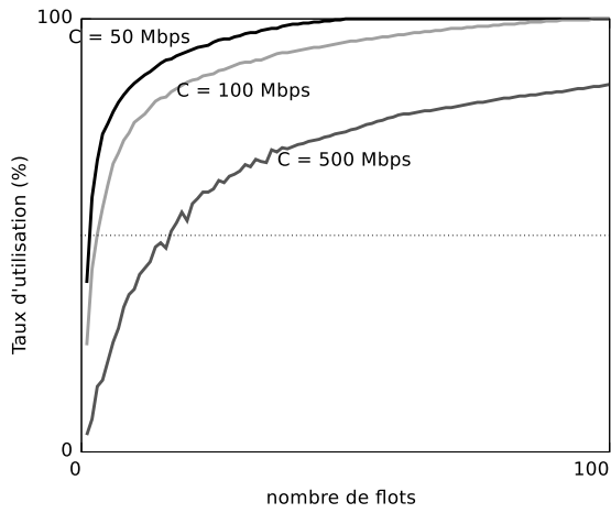
FIGURE 4.10 – Taux d'utilisation de la capacité résiduelle \phi(i) atteint pour chaque nombre i de flots en cours ; et espérance du débit \gamma d'un flot en fonction de la charge \rho , pour différentes capacités de lien
