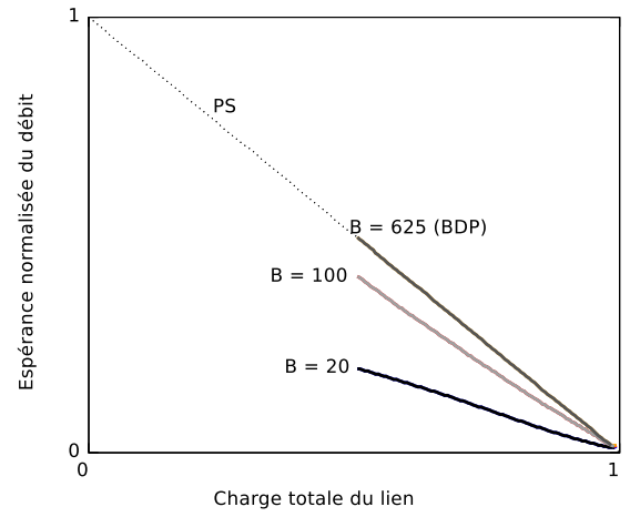
FIGURE 4.9 – Taux d'utilisation de la capacité résiduelle \phi(i) atteint pour chaque nombre i de flots en cours ; et espérance du débit \gamma d'un flot en fonction de la charge \rho , pour différentes tailles de buffer
