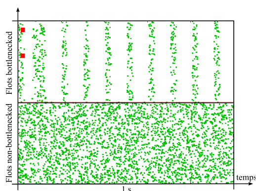
FIGURE 4.6 – Représentation des arrivées de paquets TCP NewReno sur un lien avec un buffer de 20 paquets. Chaque point est un paquet ; sa position verticale est aléatoire ; les carrés sur la gauche représentent des paquets perdus.
