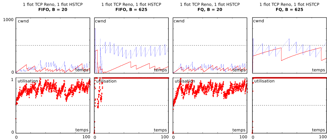
FIGURE 5.7 – Evolution de cwnd et utilisation de la bande passante disponible faite par un flot TCP Reno en compétition avec un flot HSTCP, en compétition avec une charge background de 50%. Le lien est respectivement FIFO (les deux figures de gauche) et FQ (les deux figures de droite), et les tailles de buffer considérées sont de 20 et 625 paquets.
