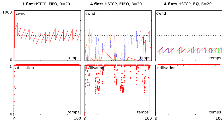
FIGURE 5.9 – Evolution de cwnd et utilisation de la bande passante disponible par 1 flot (à gauche) et 4 flots HSTCP (au milieu) sur un lien FIFO, et par 4 flots HSTCP sur un lien FQ (à droite). Les flots sont en compétition avec une charge background de 50%, et la taille de buffer considérée est de 20 paquets.
