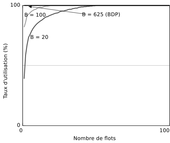
FIGURE 4.9 – Taux d'utilisation de la capacité résiduelle \phi(i) atteint pour chaque nombre i de flots en cours ; et espérance du débit \gamma d'un flot en fonction de la charge \rho , pour différentes tailles de buffer
