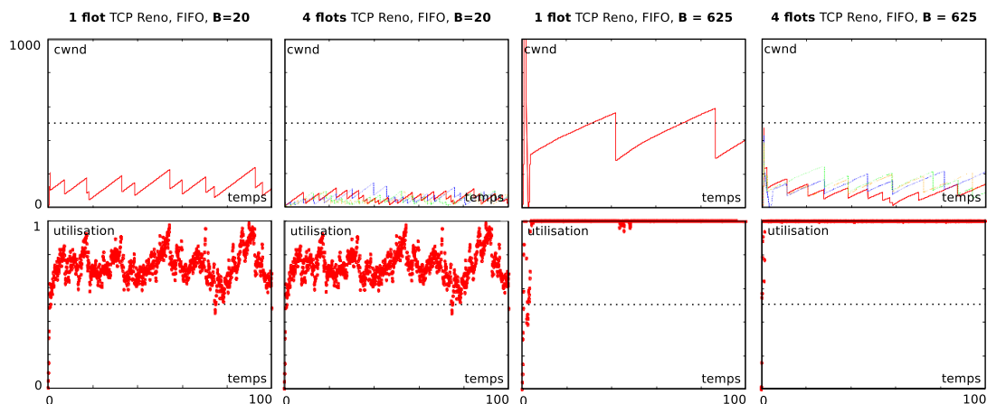
FIGURE 5.8 – Evolution de cwnd et utilisation de la bande passante disponible faite par 1 et 4 flots TCP Reno en compétition avec une charge background de 50%. Le lien est FIFO, et les tailles de buffer considérées sont de 20 paquets (les deux figures de gauche) et 625 paquets (les deux figures de droite).
