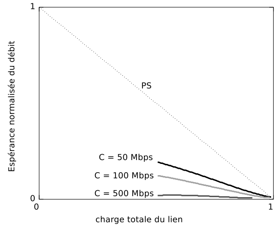
FIGURE 4.10 – Taux d'utilisation de la capacité résiduelle \phi(i) atteint pour chaque nombre i de flots en cours ; et espérance du débit \gamma d'un flot en fonction de la charge \rho , pour différentes capacités de lien
