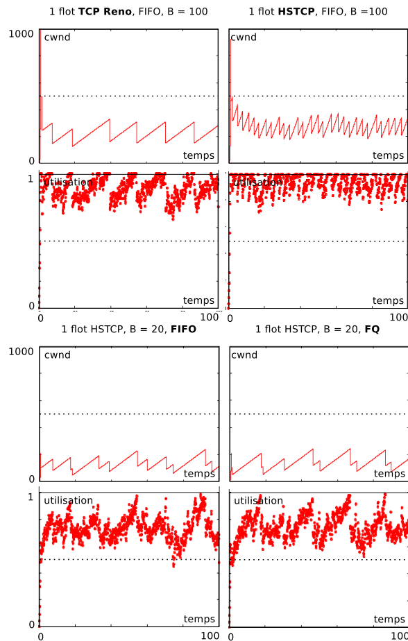
FIGURE 5.5 – Evolution de cwnd et utilisation de la bande passante disponible faite par une connexion TCP Reno et une connexion HSTCP en compétition avec une charge background de 50%, dans des scénarios FIFO et FQ impliquant plusieurs tailles de buffer.
